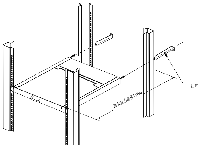
图 2-1 机架安装图(一)
