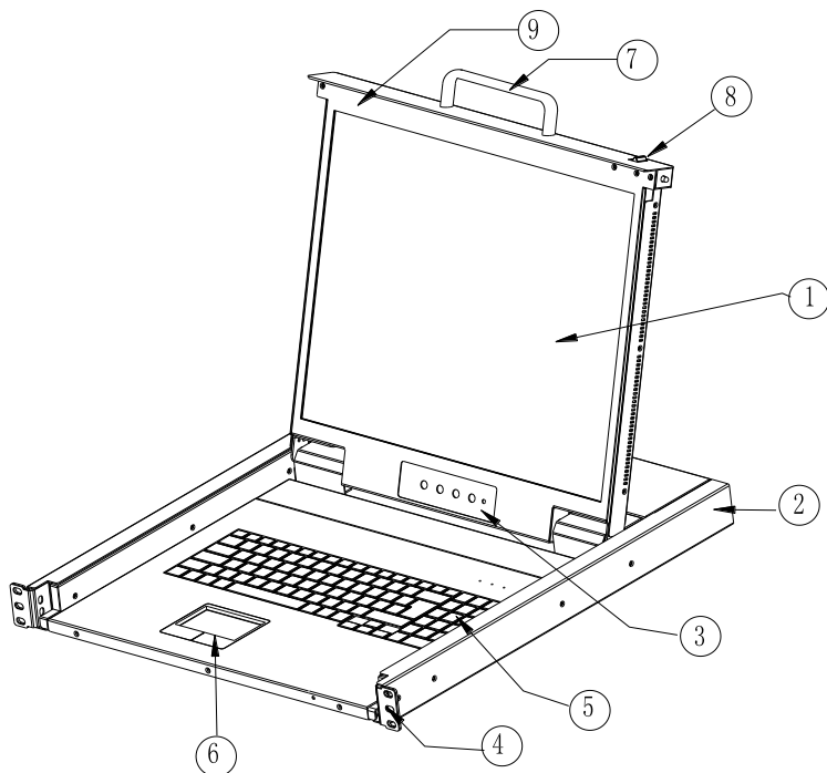
图 1-2 前视图
