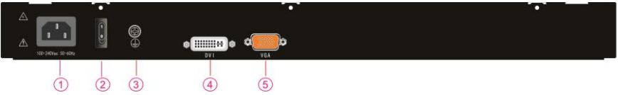
图 3-1 后视图
