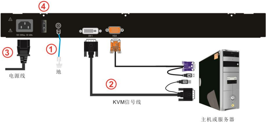
图 3-2 连线方式
